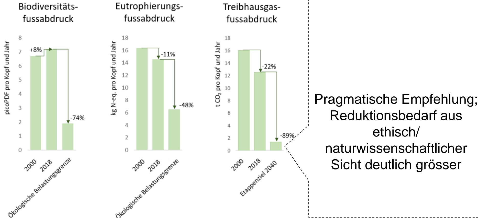
Abbildung 4 Entwicklung der Umweltfussabdrücke pro Person zwischen 2000 und 2018 und der weitere Reduktionsbedarf
