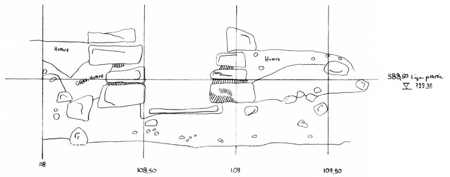
Grab 102, Profil (Grabungszeichnung)
