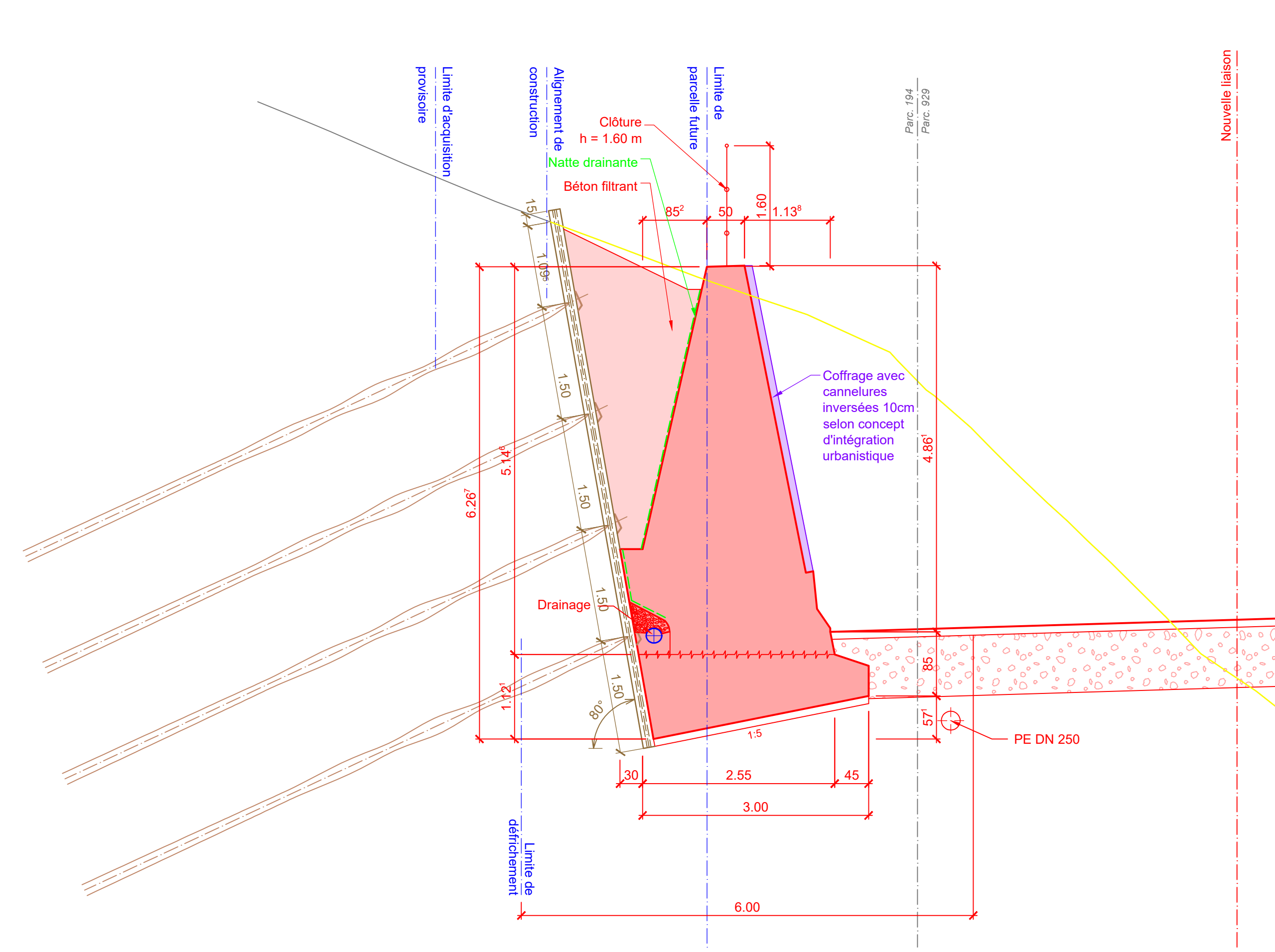
Coupe 2-2 1:50 Section B km 0+270
