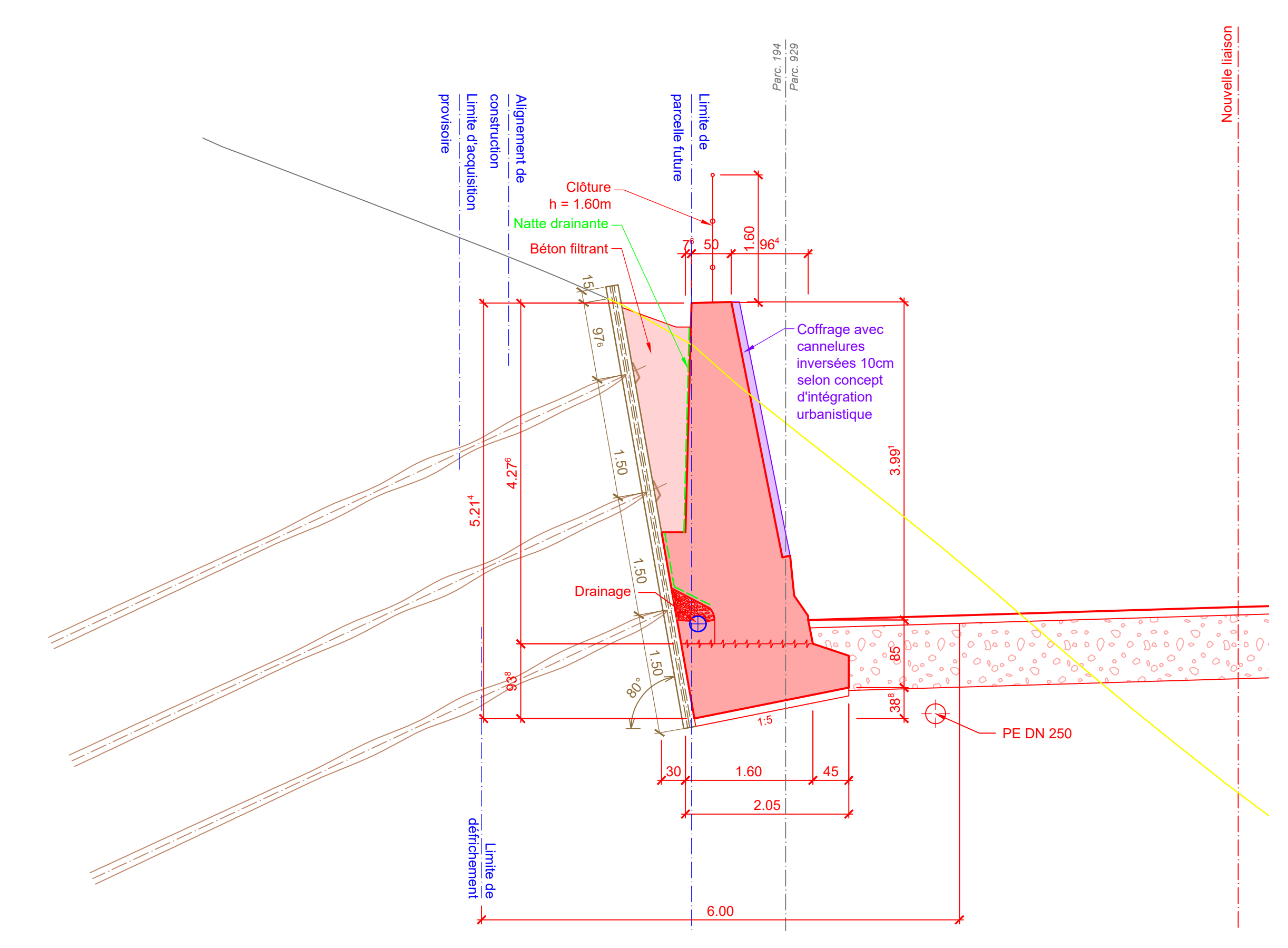
Coupe 1-1 1:50 Section A km 0+250
