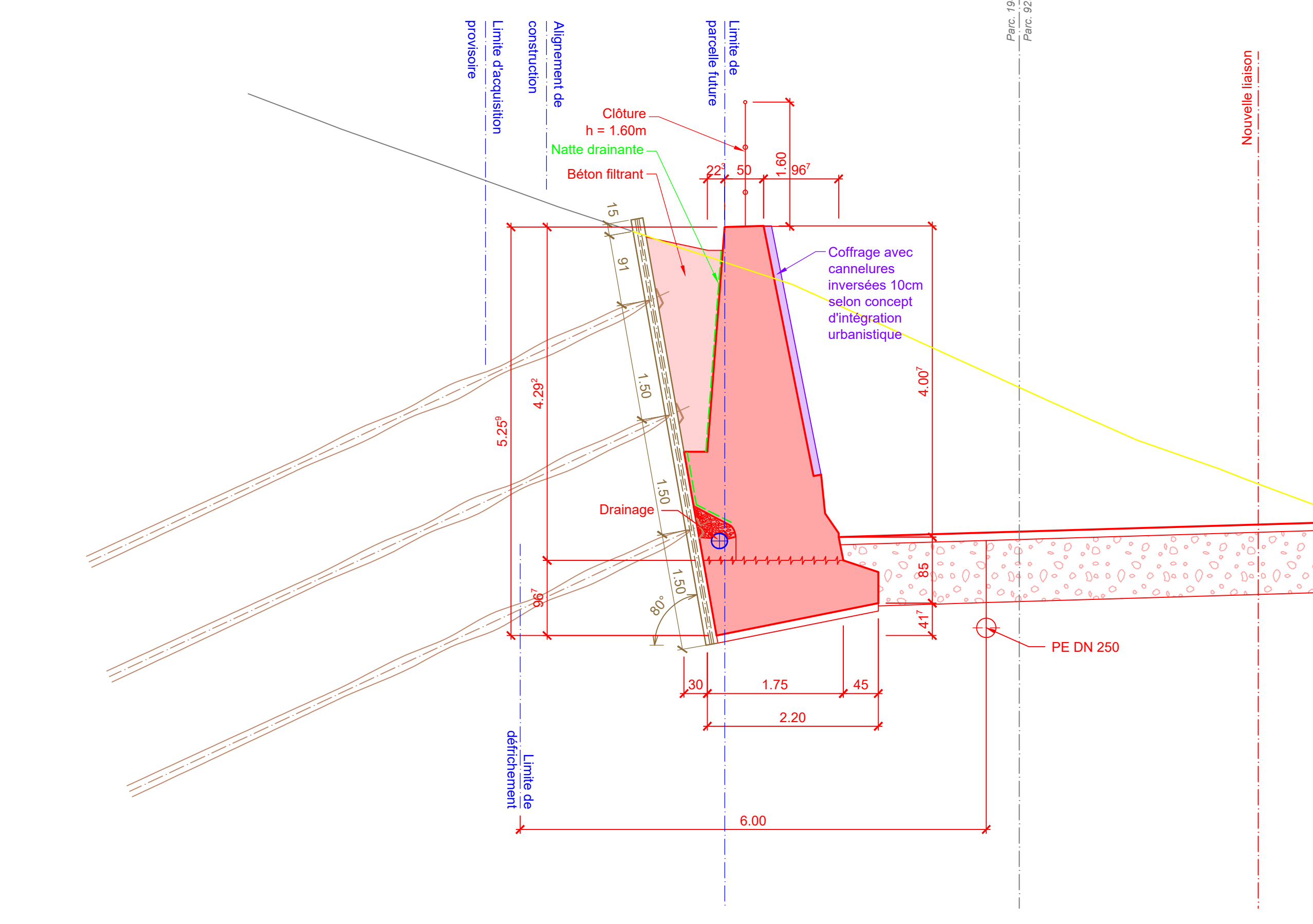
Coupe 3-3 1:50 Section C km 0+330
