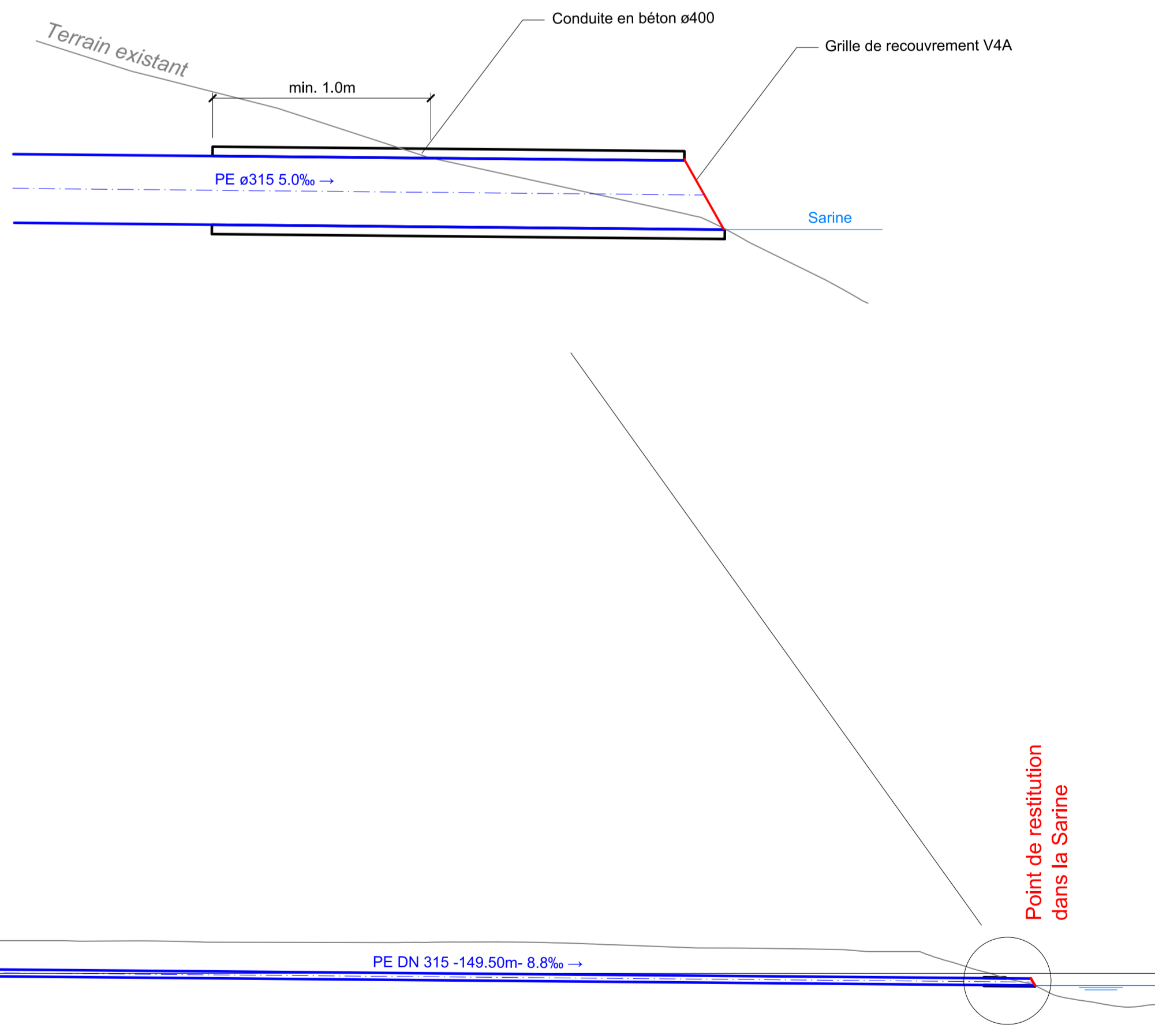
Plan de détail 1:20 Exutoire dans la Sarine
