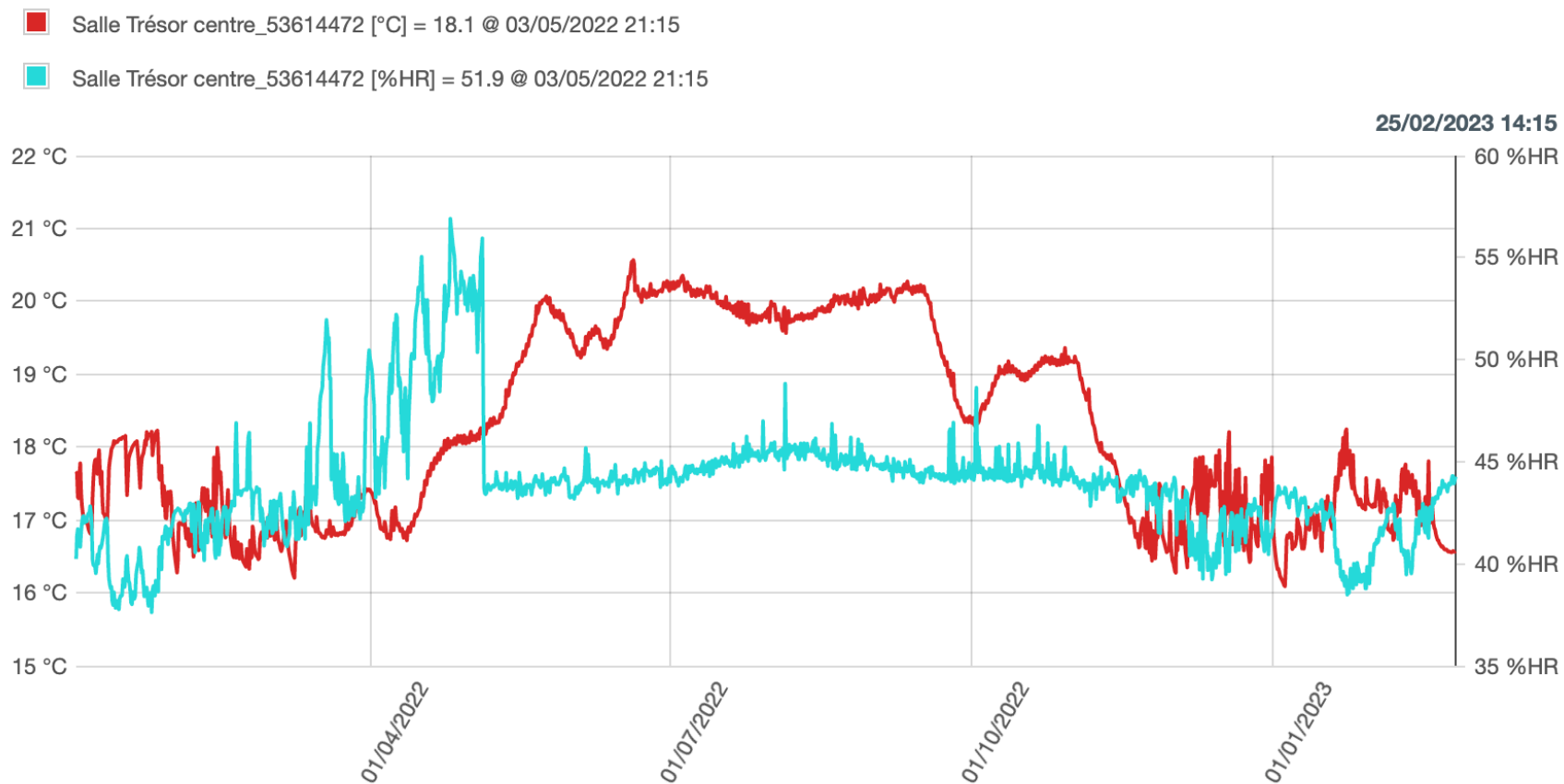
Mesures thermo-hygro-métriques de la vitrine de la Grande châsse avec des valeurs peu satisfaisantes malgré une centrale climatique
