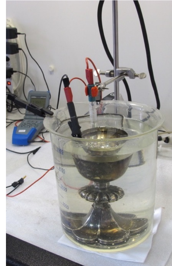
Traitement par électrolyse en immersion d'une coupe en argent avec col doré (XVe) Paroisse de Daillens (VD)
